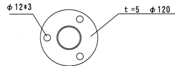
V-スプレット詳細
