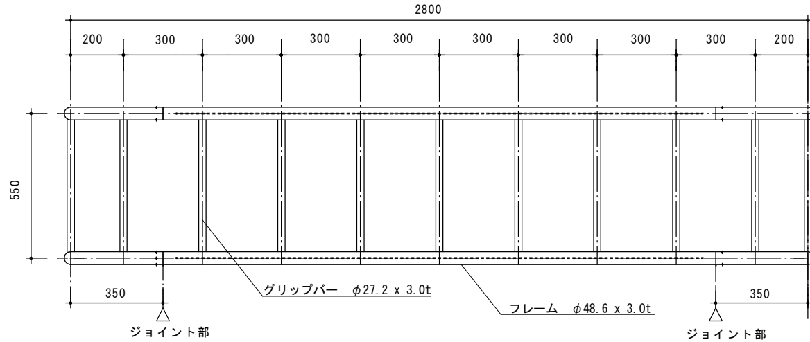
平面図
