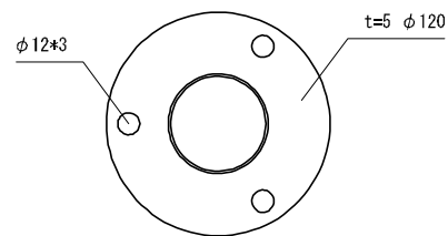
ベースプレート詳細
